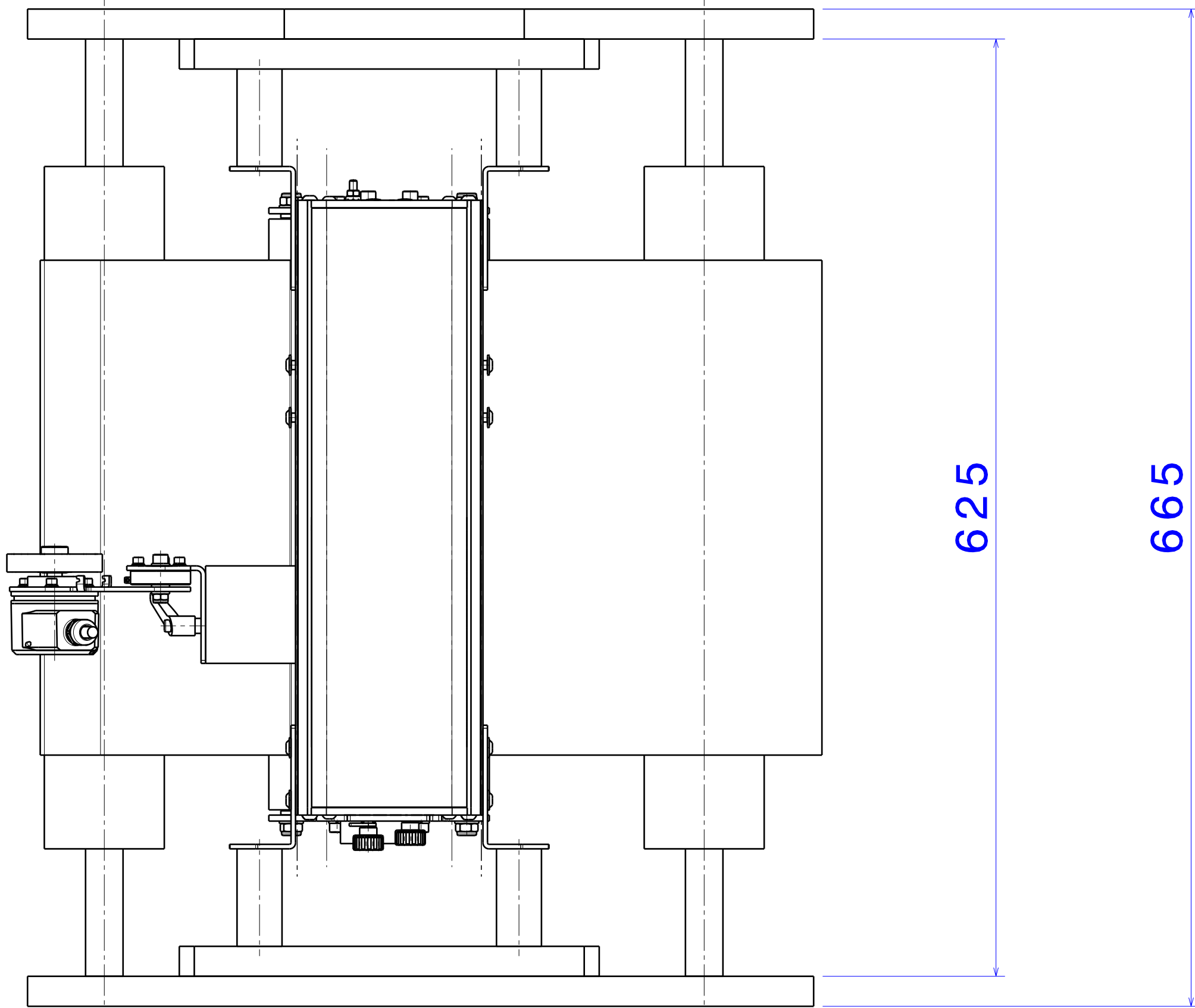
Vue de dessus Echelle : 1:3
