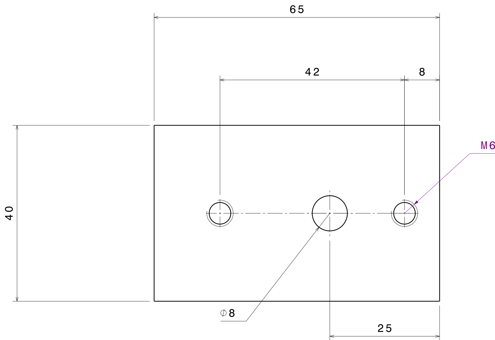
Vue de face Echelle : 2:1
