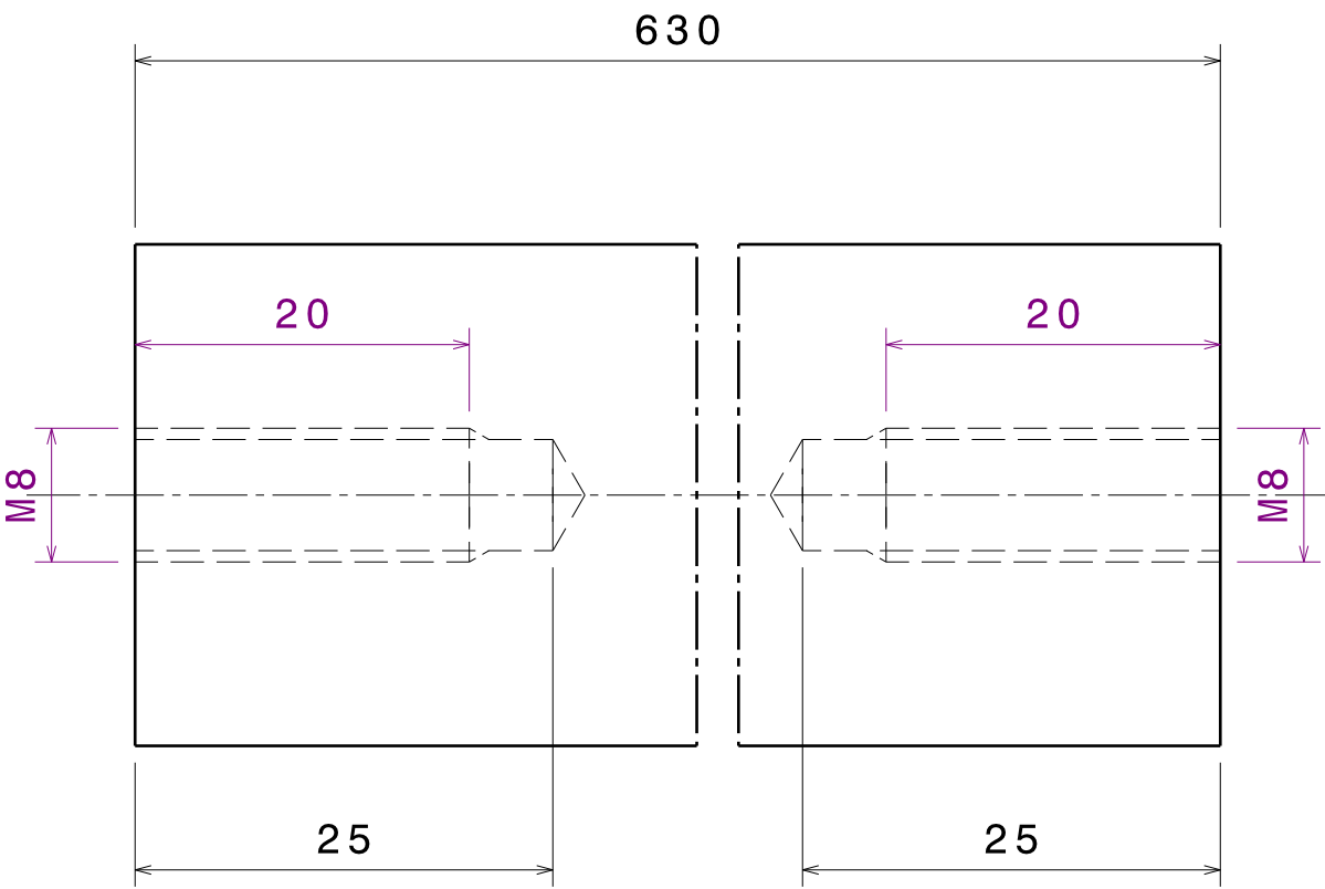
Vue de gauche Echelle : 2:1
