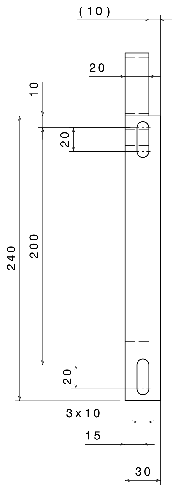
Vue de face Echelle : 1:2
