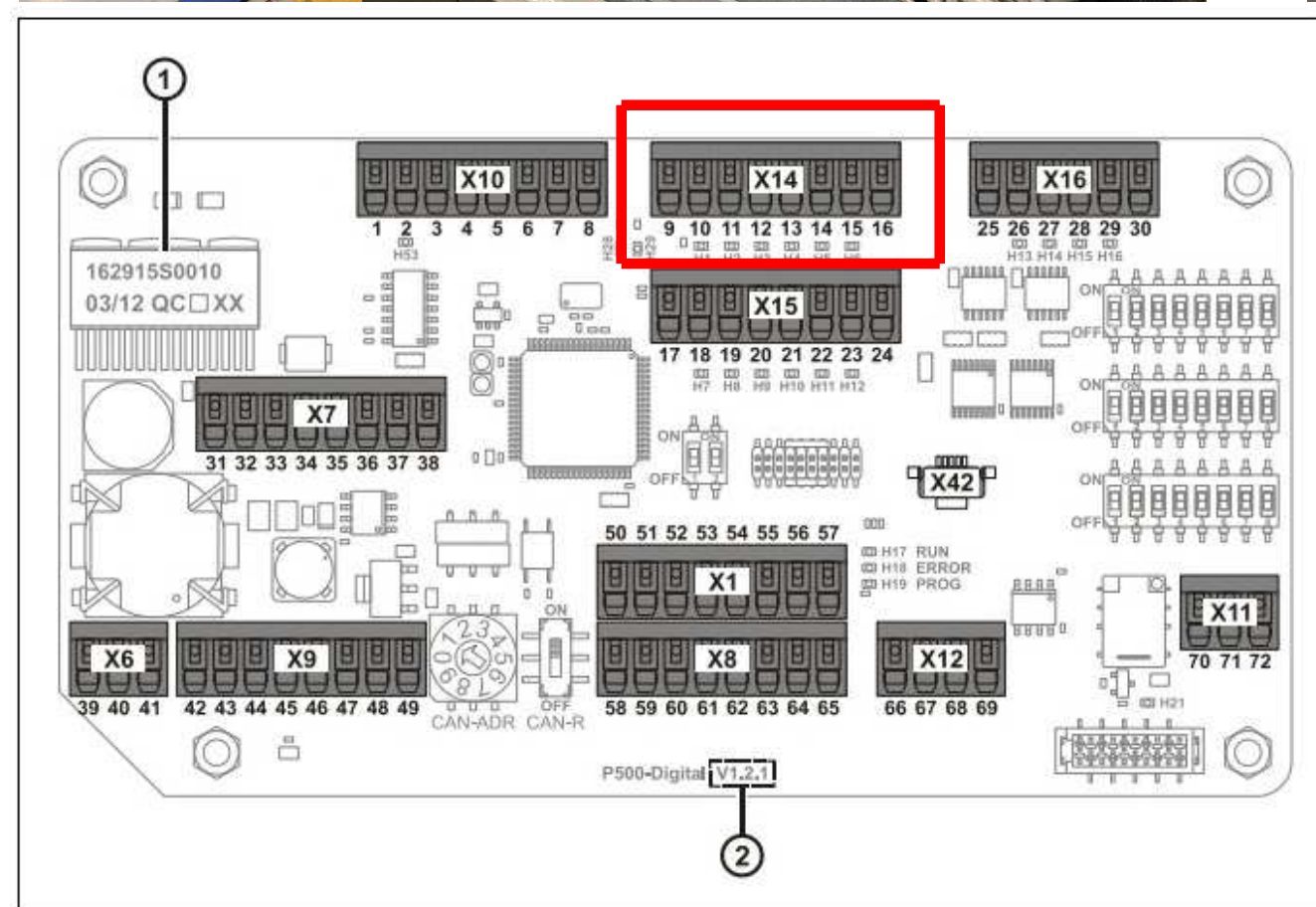
7.8.10 Terminal Strip X14 - Digital Inputs 1...6, EFE 1000
