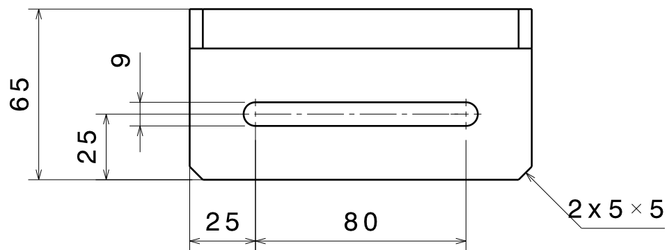
Vue de dessus Echelle : 1:2
