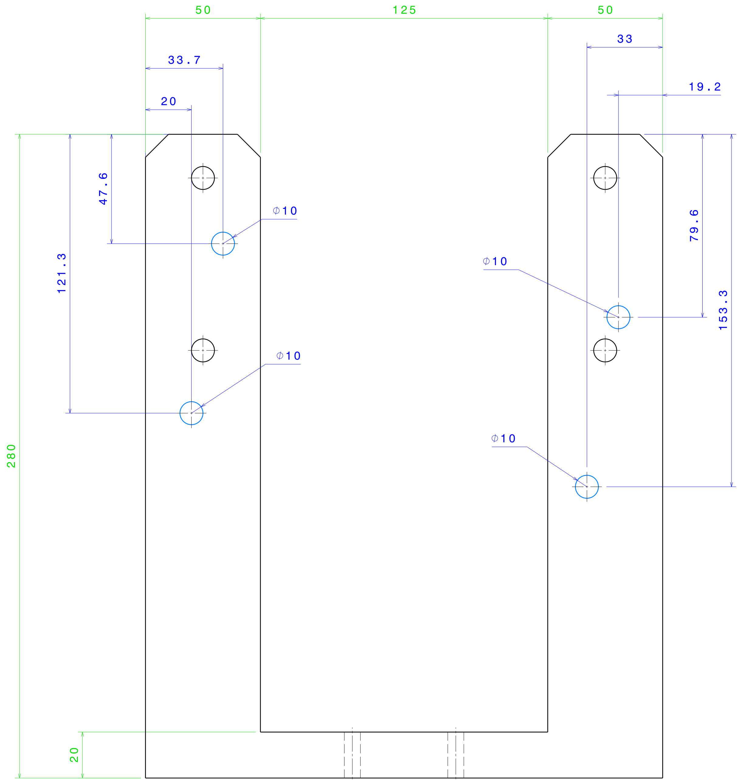
Vue de face Echelle : 1:1
