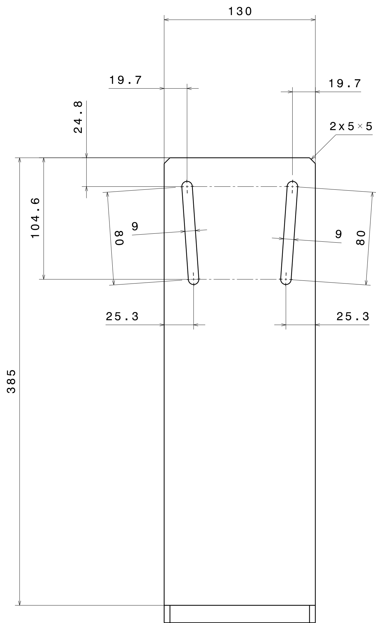
Vue de face Echelle : 1:2
