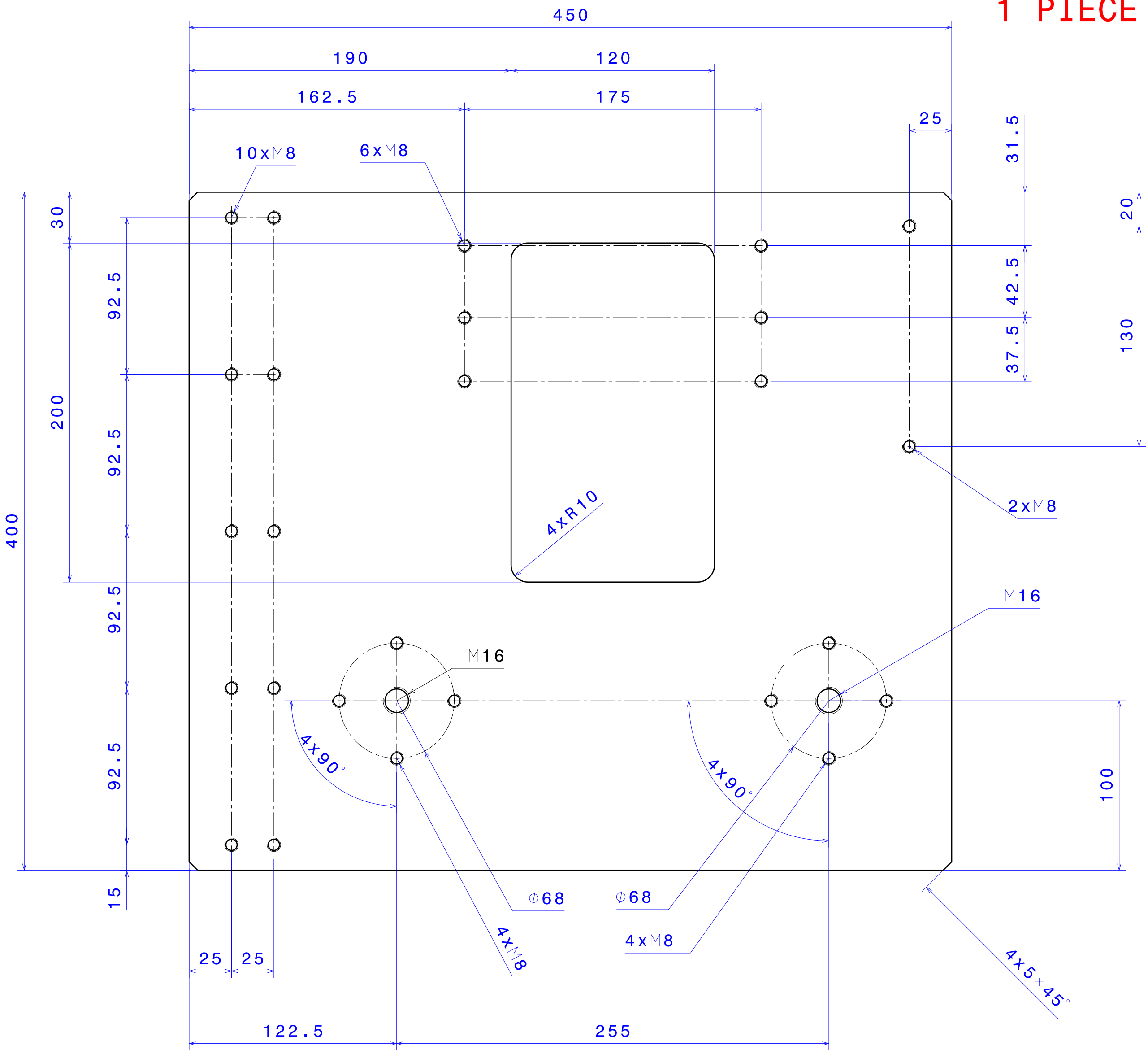
Vue de face Echelle : 1:2
