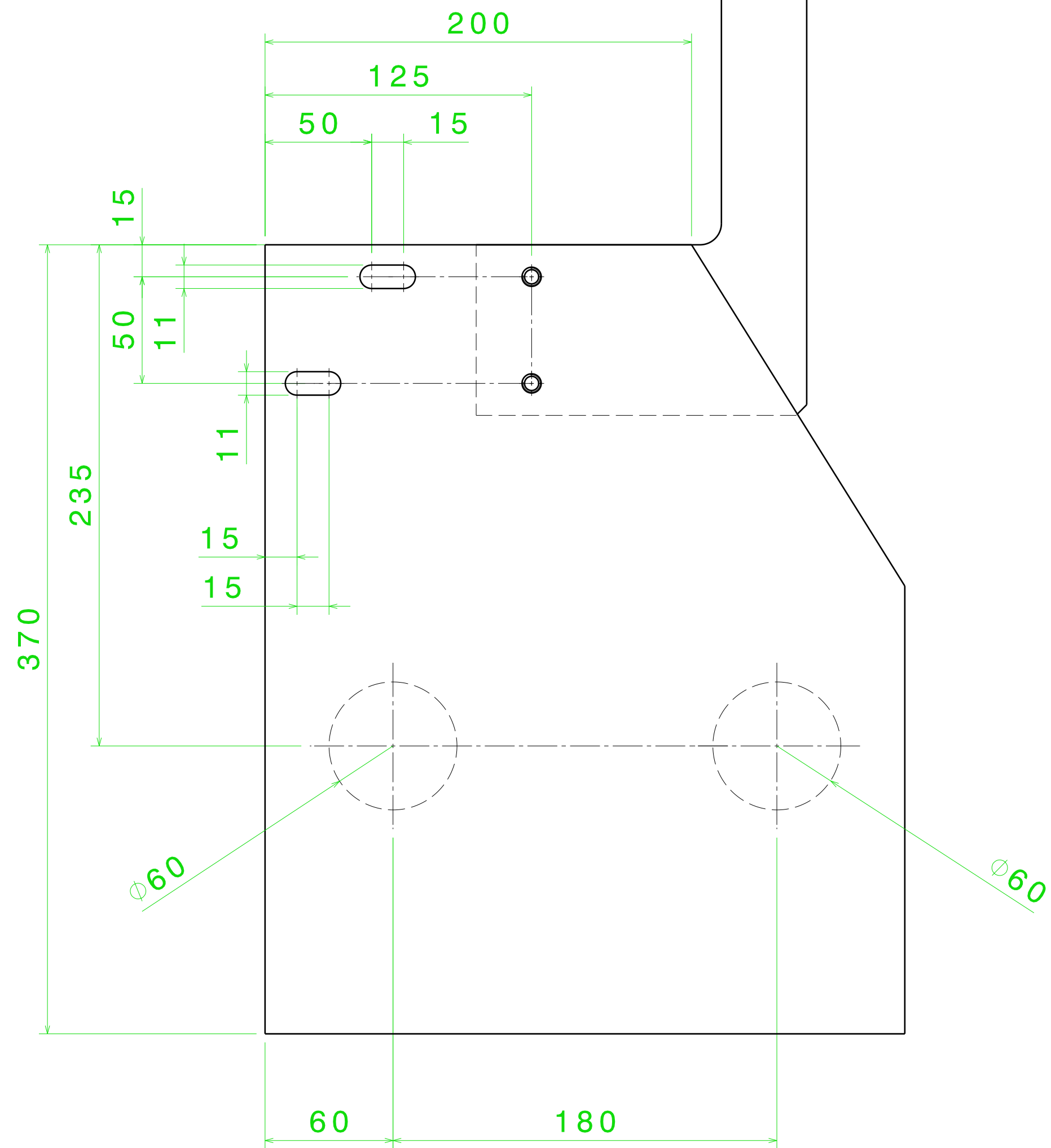
Vue de face Echelle : 1:2
