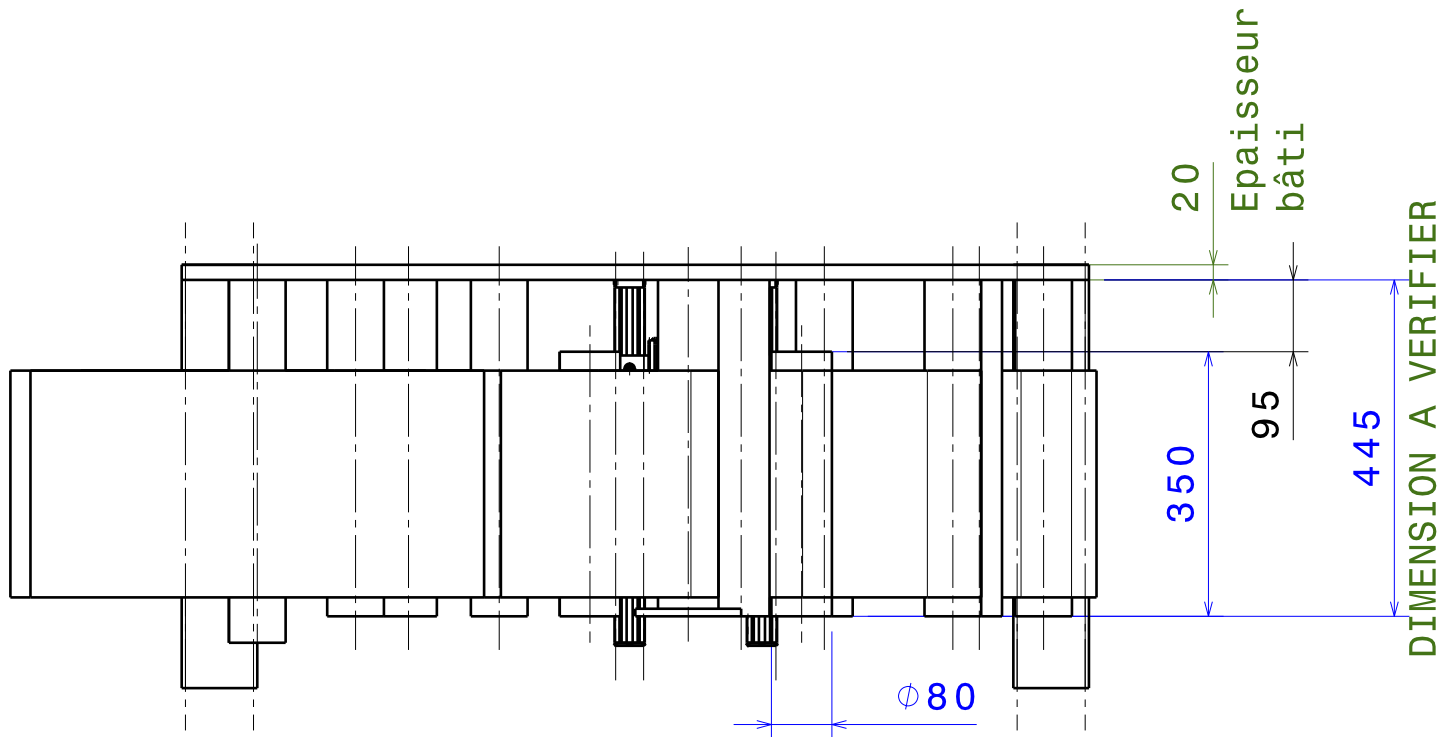
Vue de dessus Echelle : 1:10
