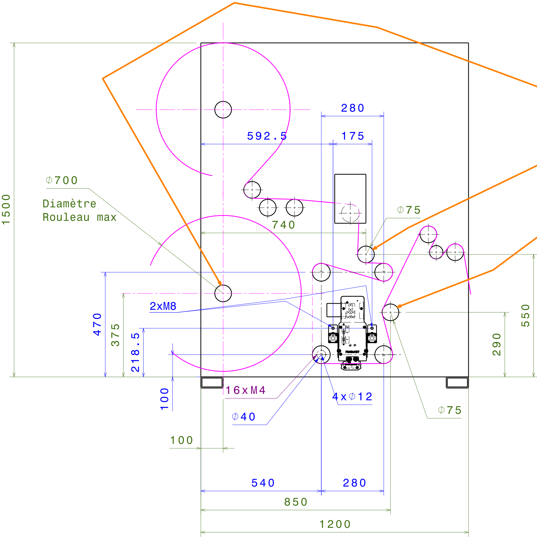
Vue de face Echelle : 1:10
