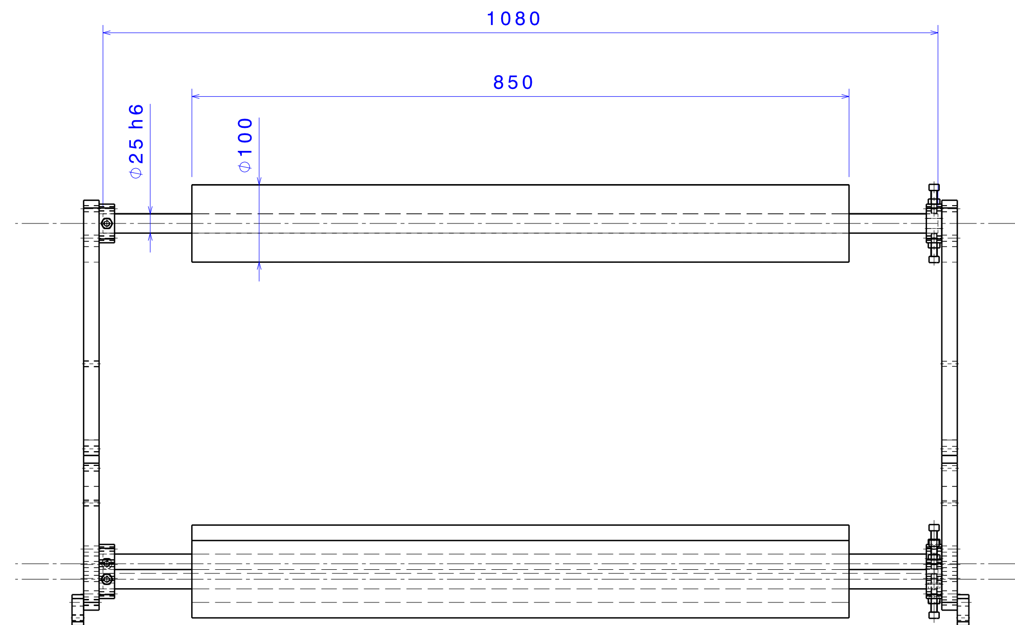
Vue de face Echelle : 1:5
