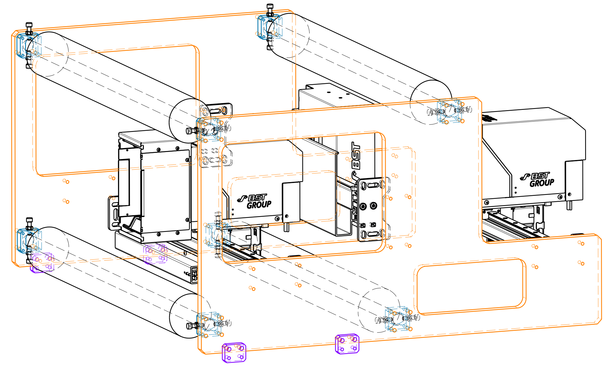
Vue isométrique Echelle : 1:5
