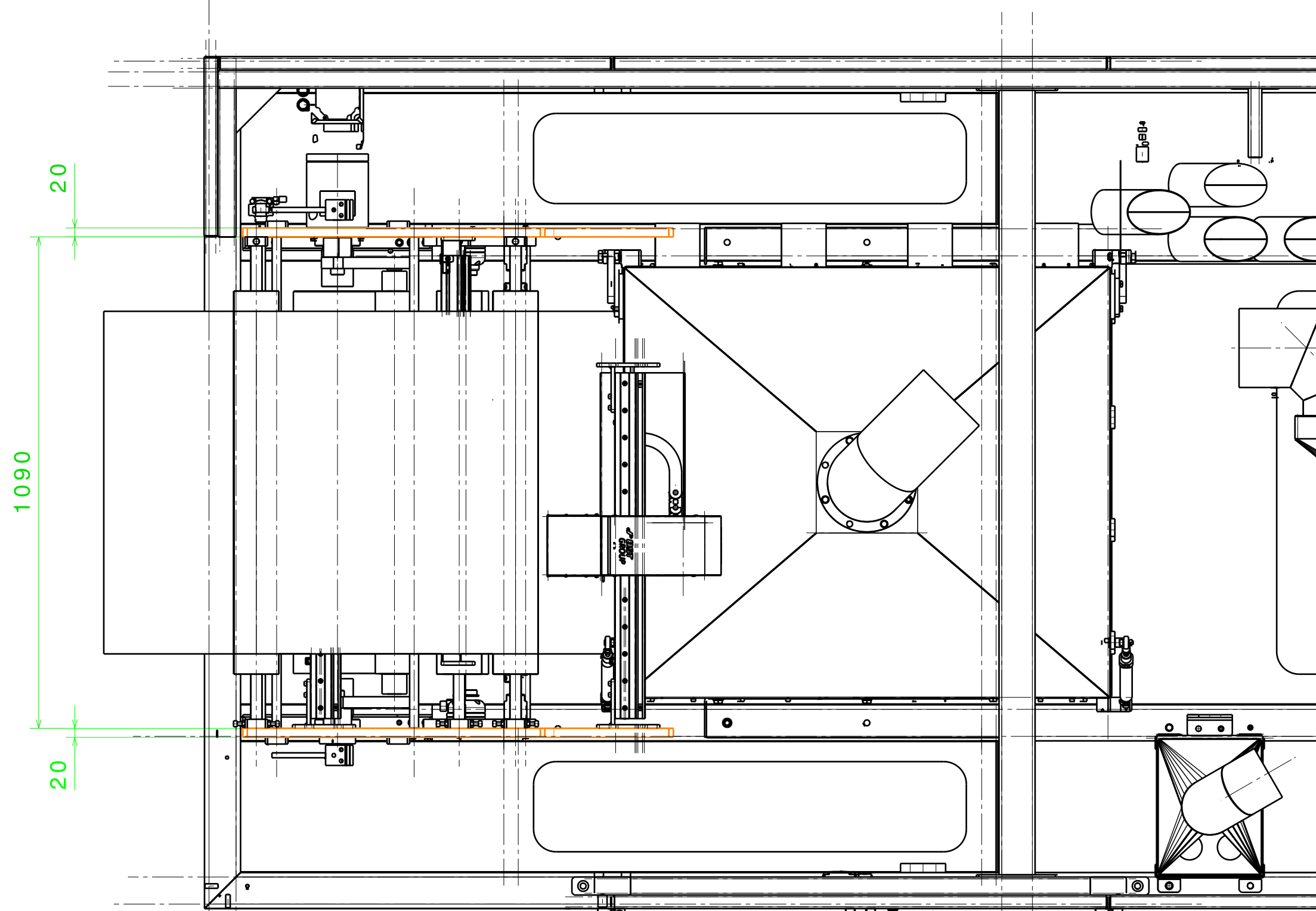
Vue de dessus Echelle : 1:10
