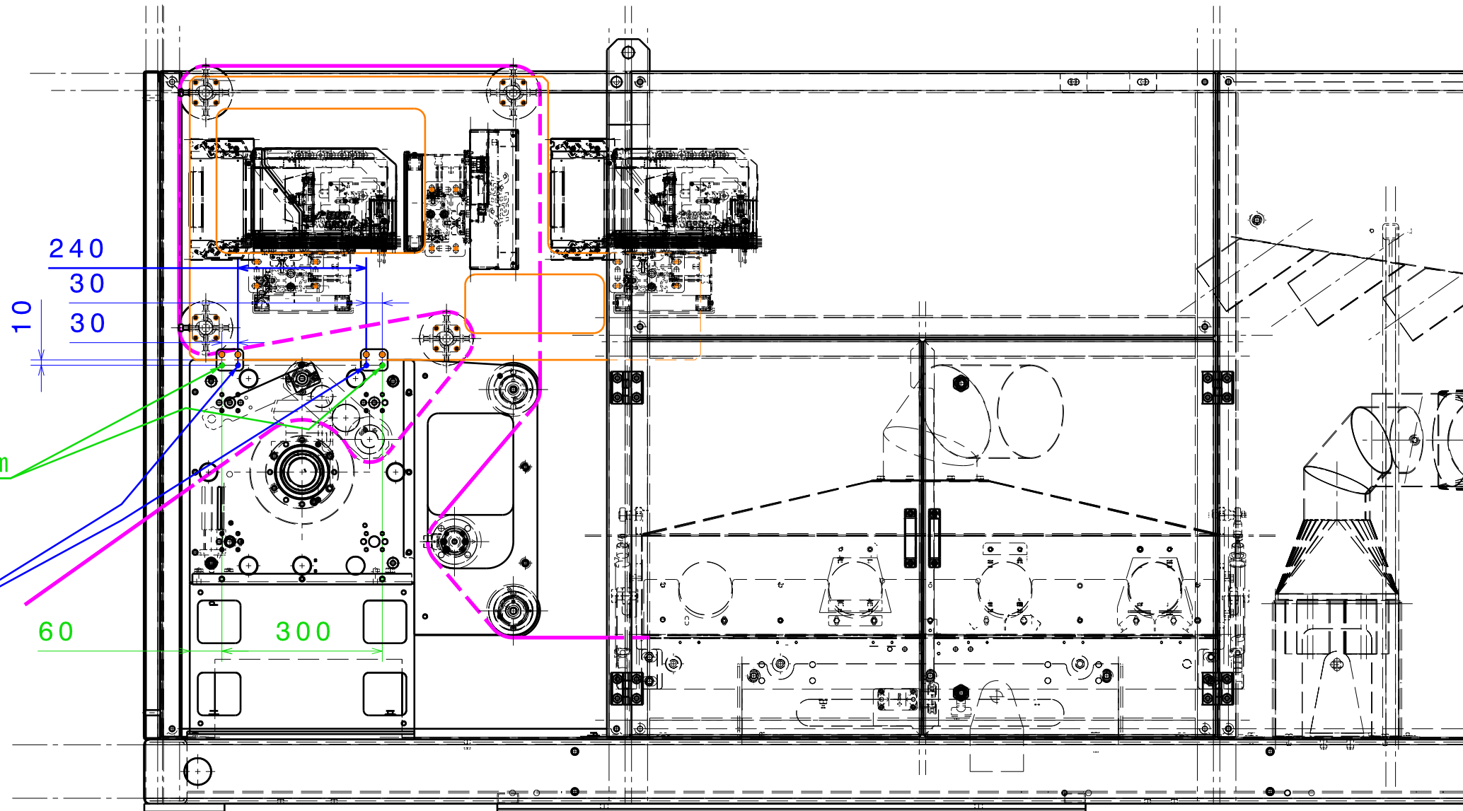
Vue de face Echelle : 1:10
