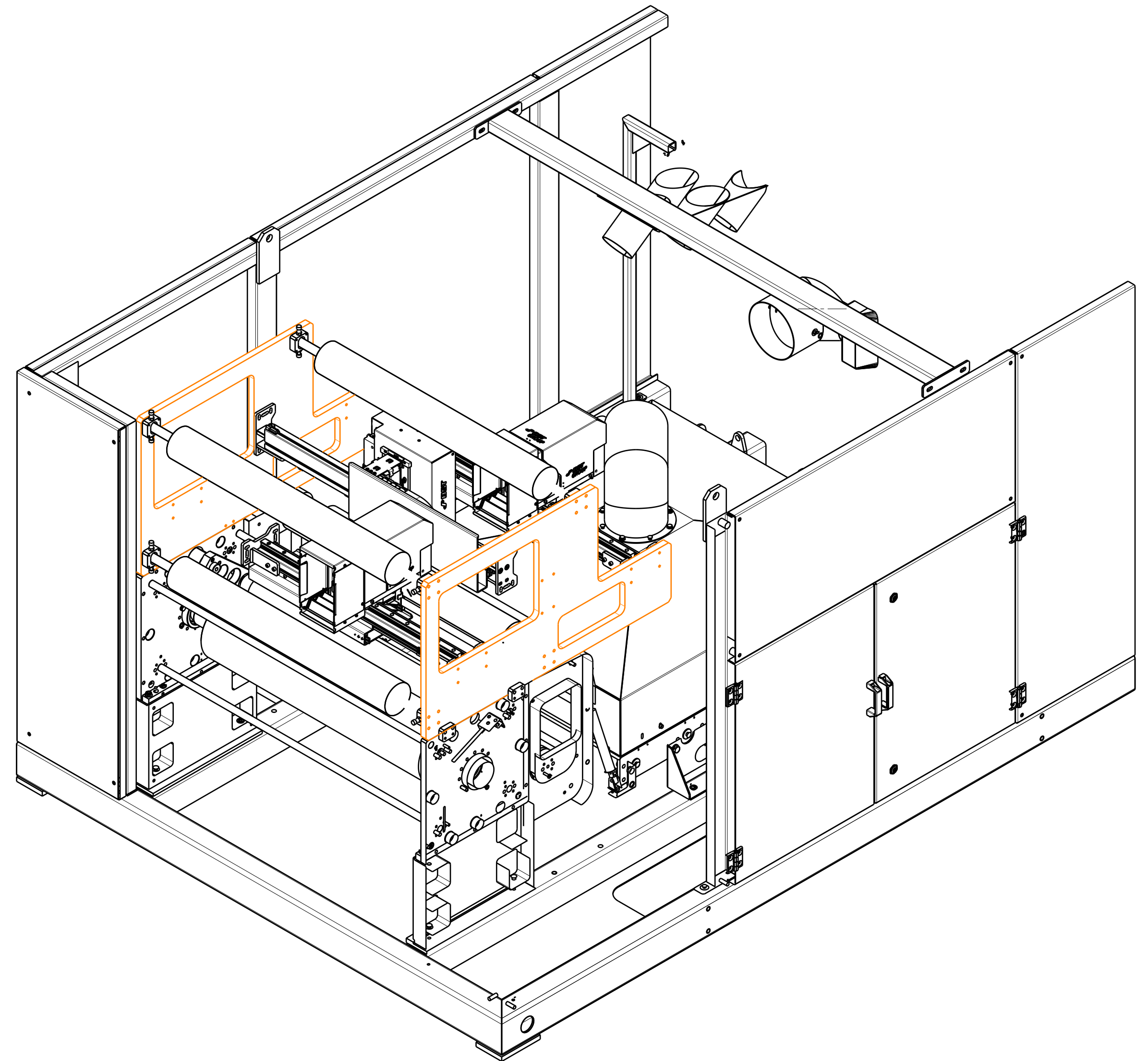
Vue isométrique Echelle : 1:10
