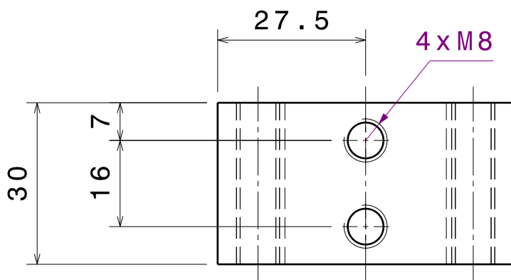
Vue de dessus Echelle : 1:1
